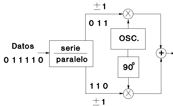
Figura 1.21 Modulador QPSK.
