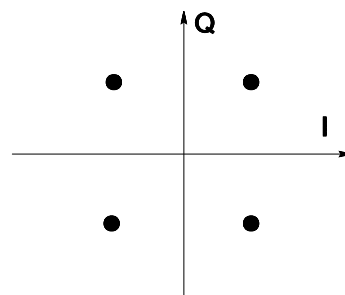
Figura 1.20 Constelación QPSK.
